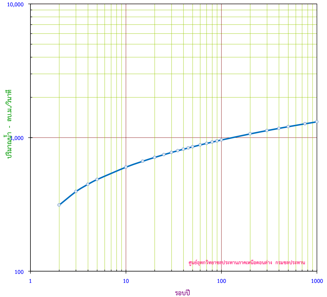
กราฟแสดง ปริมาณน้ำสูงสุดรายปี ขนาดรอบปีต่างๆ สถานี W.4A อ.คลองขลุง จ.กำแพงเพชร
